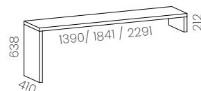
MTV3 - N / MTV4 - N / MTV5 - N (L, D)
